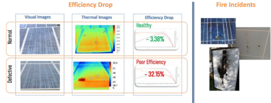
ภาพเปรียบเทียบการทำงานของกล้องถ่ายภาพความร้อนและการตรวจจับแผงที่เกิดปัญหาได้อย่างแม่นยำ
