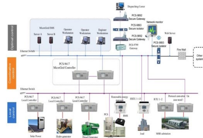
ภาพแสดงผังระบบควบคุมไฟฟ้าอัจฉริยะโครงการพัฒนาระบบไฟฟ้าแบบโครงข่ายไฟฟ้าขนาดเล็กมาก (microgrid) อ.แม่สะเรียง จ.แม่ฮ่องสอน ของการไฟฟ้าส่วนภูมิภาค
